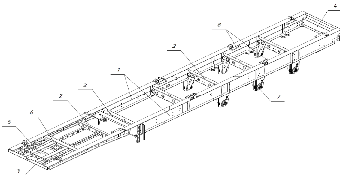
Рис. 1.4 - Рама полуприцепа
