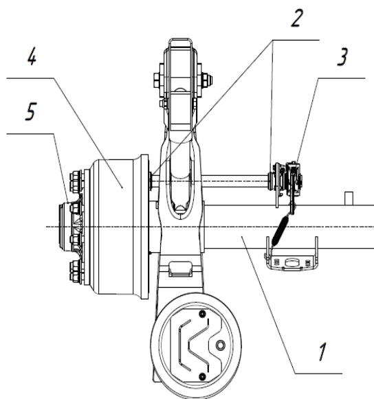
а) барабанная ось
