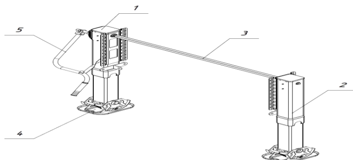
Рис. 2.12 – Опорное устройство
