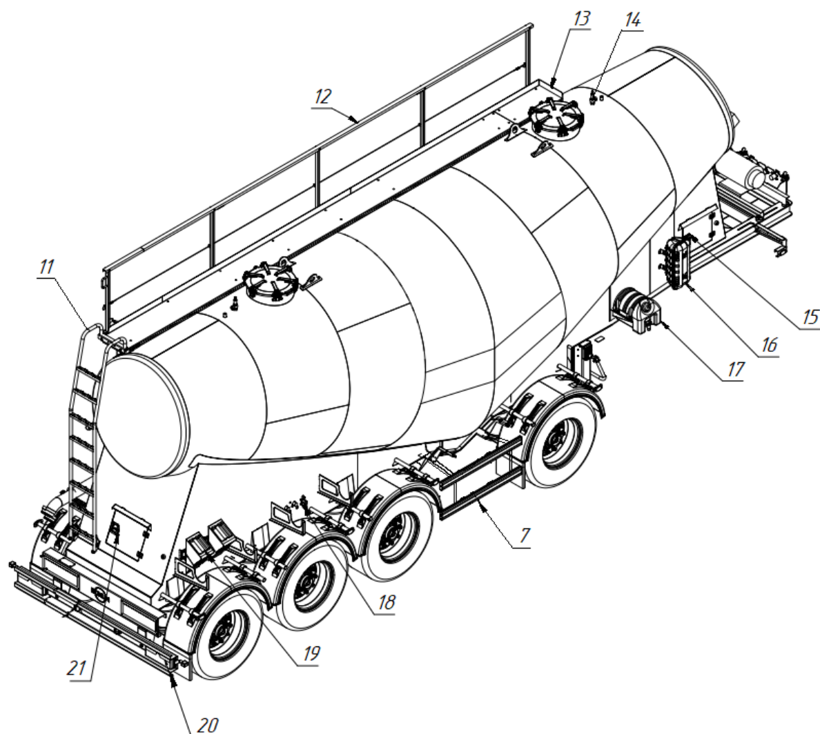
Рис. 2.2 вариант 2 - общий вид полуприцепа типа 914211 модификации 914231
