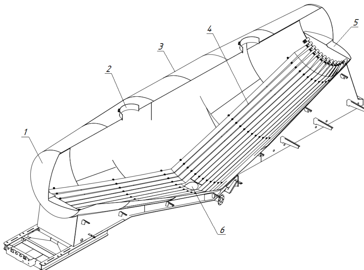
Рис. 2.3 – Колба полуприцепа
