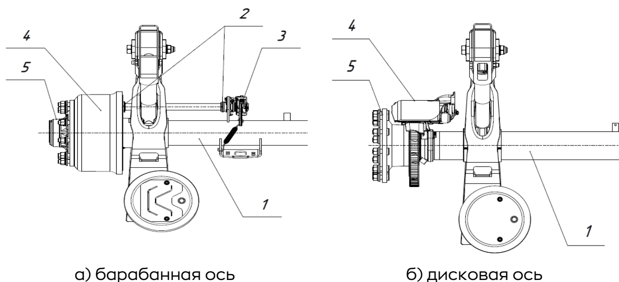
Рис. 2.5 - Оси
