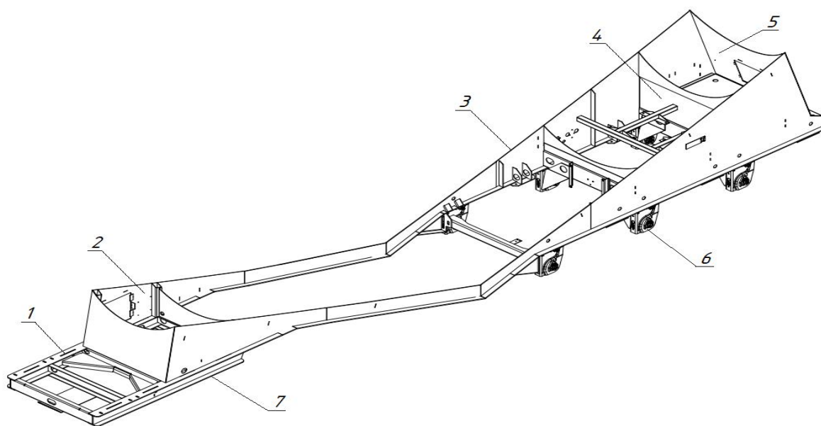
Рис. 2.4 - Рама полуприцепа
